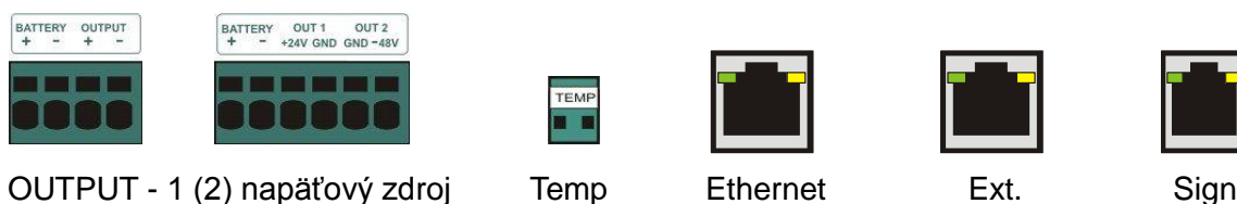
Obrázok 4 – Popis konektorov zdroja LS150.JS POE(8X)
