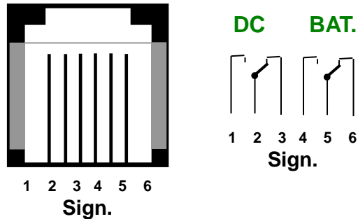
Obrázok 1 – zapojenie signalizácie zdroja LS150.JS POE(8X)
