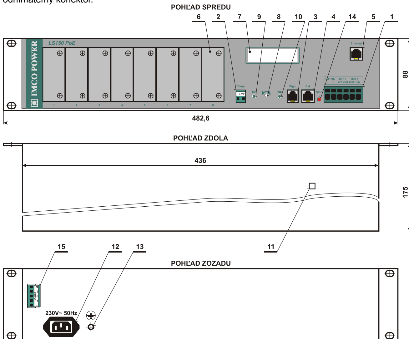
Obrázok 3 – mechanická konštrukcia zdroja LS150.JS POE(8X)
